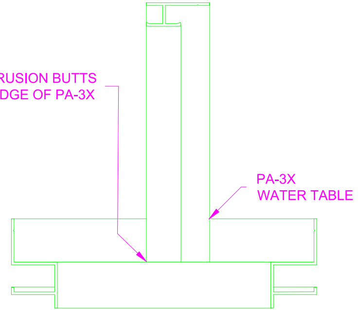
16B HORZ / VERT TERMINATION, OPTION 2
